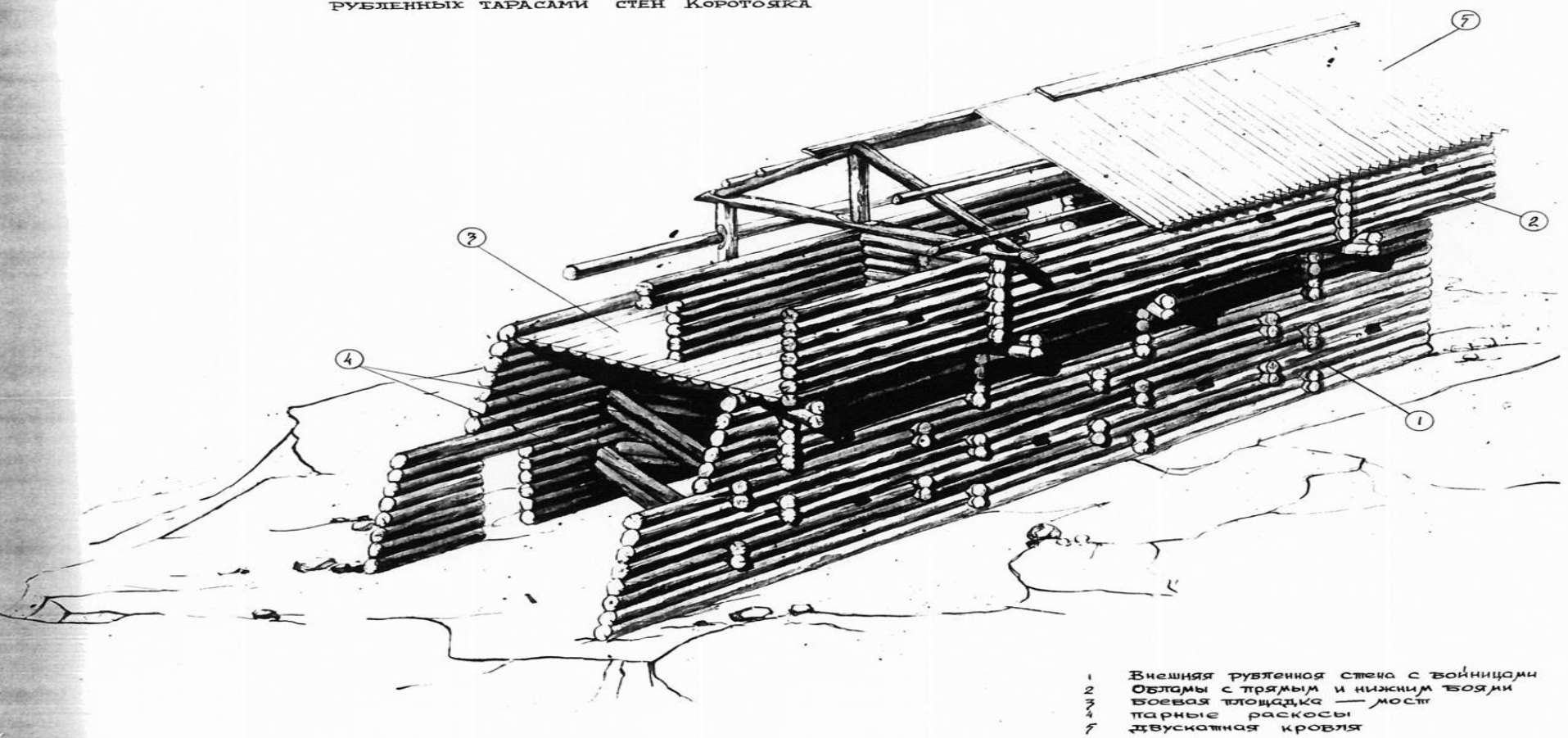
КОНСТРУКТИВНАЯ СХЕМА РУБЛЕННЫХ ТАРАСАМИ СТЕН КОРОТЮЖКА
