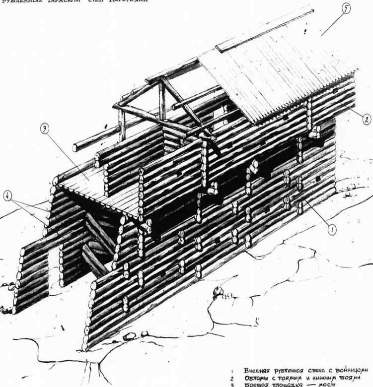
КОНСТРУКТИВНАЯ СХЕМА РУБЛЕННЫХ ТАРАСАМИ СТЕН КОРОТОЯЧКА
